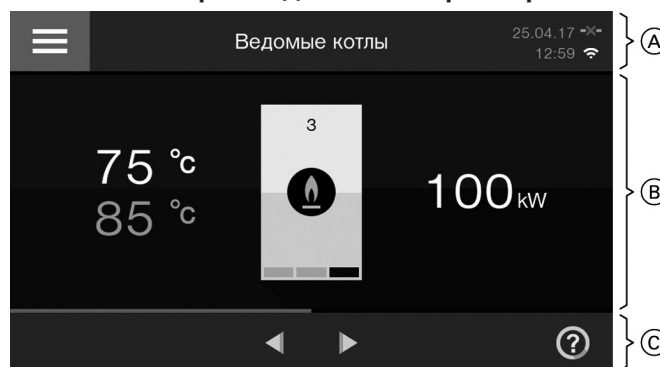
Начальный экран ведомого контроллера
