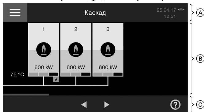
Начальный экран ведущего контроллера
